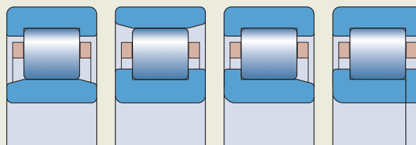
Ejemplos de configuración de pestañas guía
